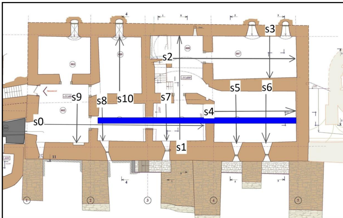
Рис. 9. Креслення цокольного поверху Палацу пристосованого під укриття [36], [3]
