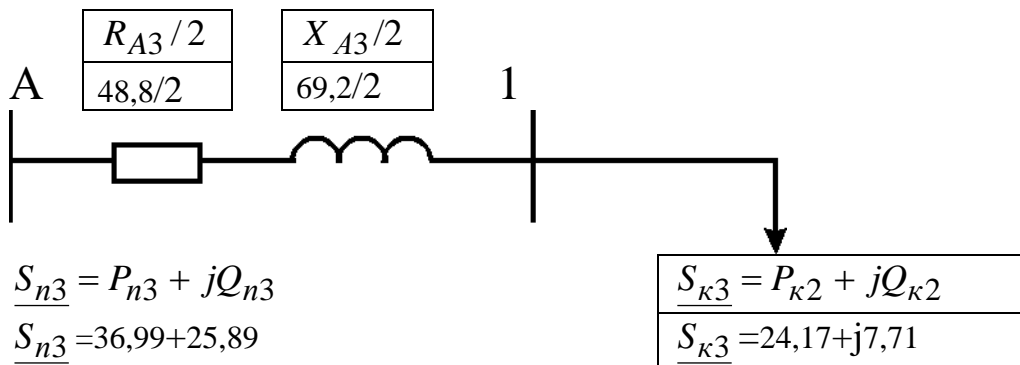
Рисунок 4.4в – Схема заміщення ділянки А-3 с приведенными навантаженнями
