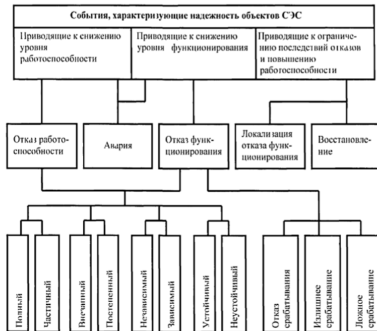
Рисунок 1.2 – Класифікація подій, що характеризують надійність об'єктів систем електропостачання
