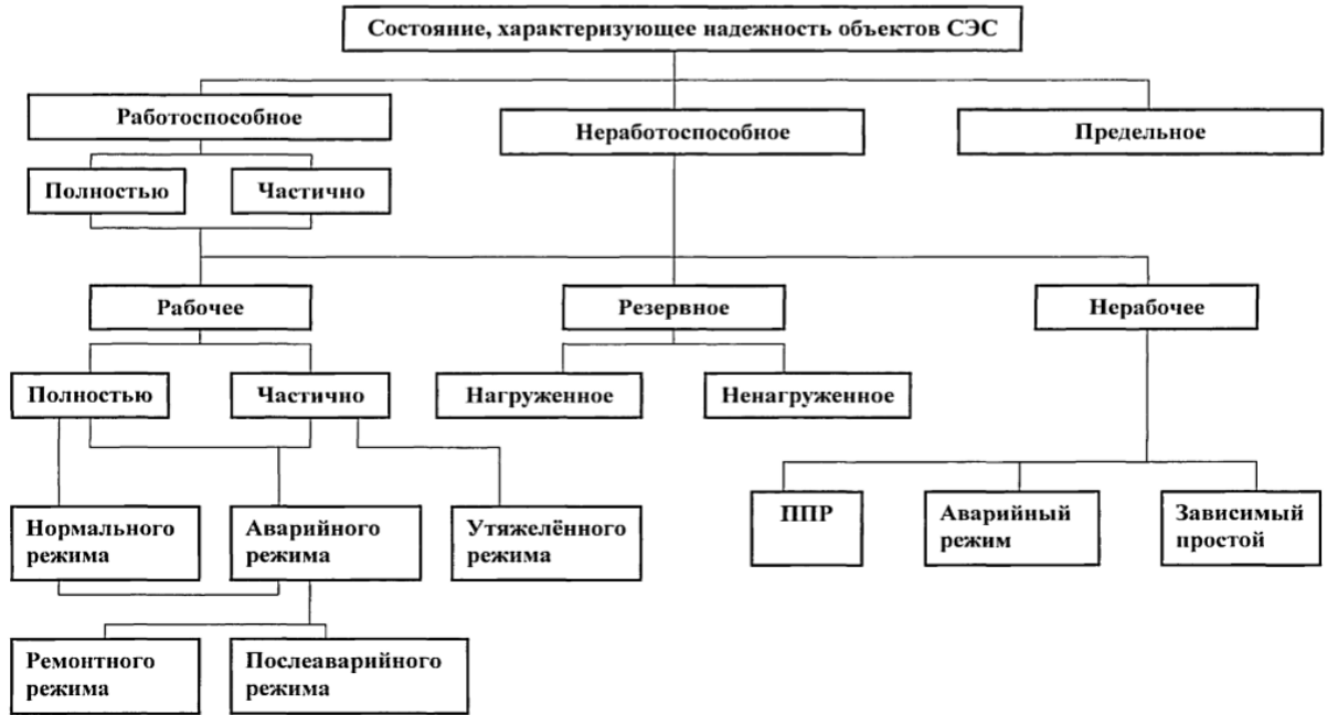
Рисунок 1.1 – Класифікація станів, що характеризують надійність об'єктів систем електропостачання НС
