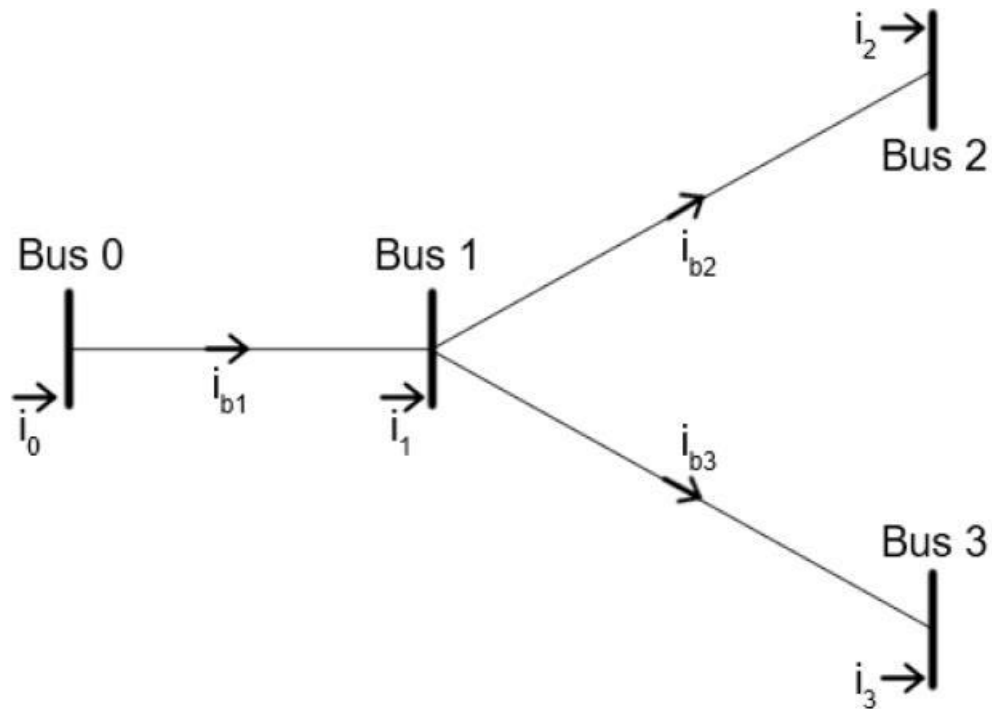
Рисунок 3.2 – Спрощена схема електромережі
