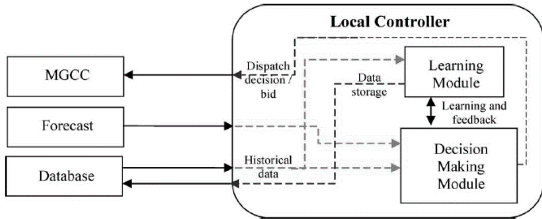
Рисунок 2.2 – Внутрішня структура системи локального керування МАСК
