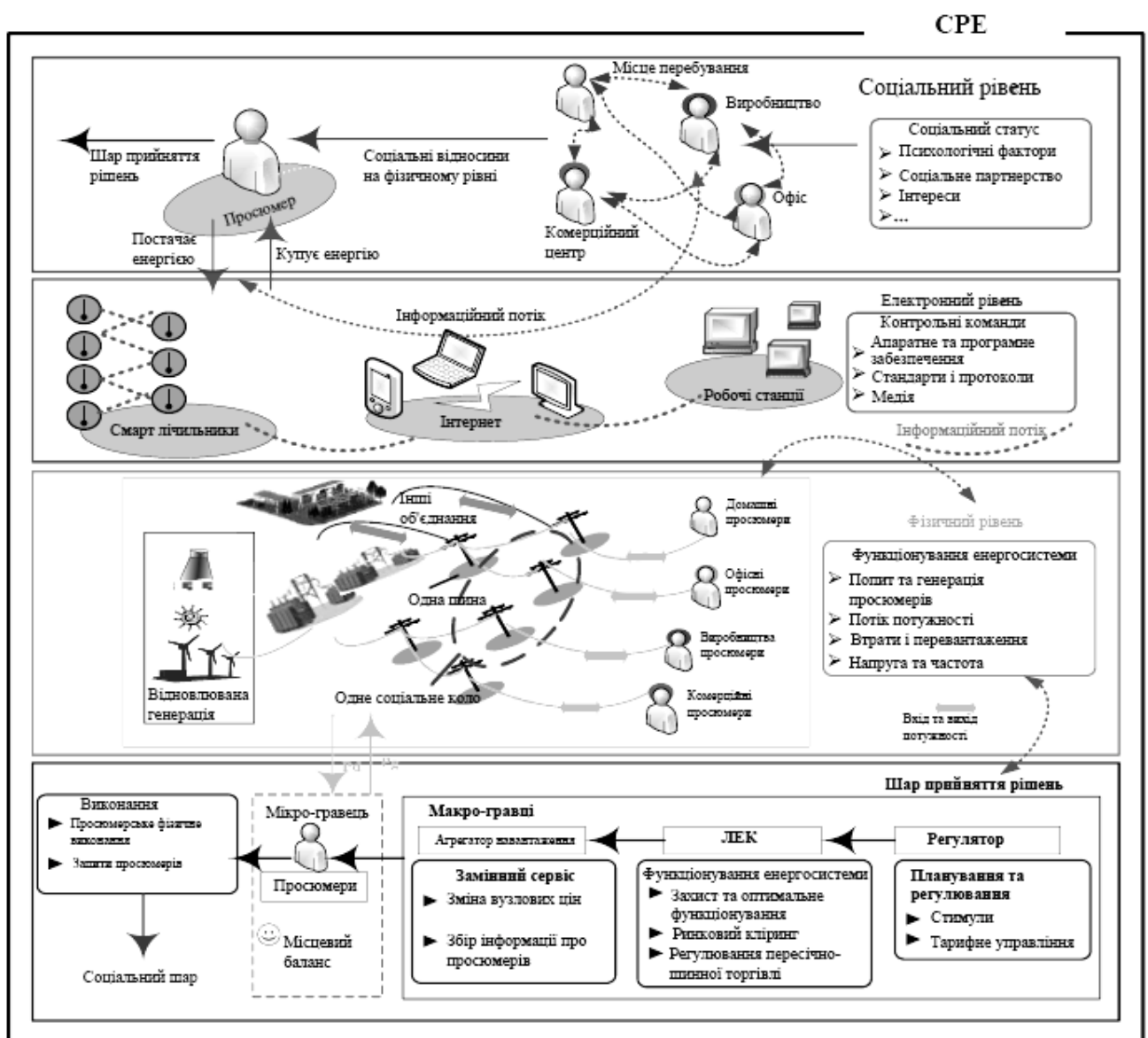
Рисунок 1.7 – Багатошарова структура симулювання для систем розподілу електроенергії
