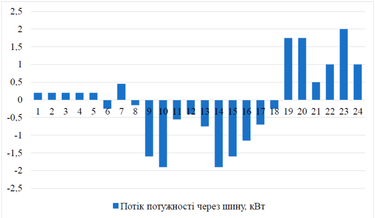
Рисунок 4.2 – Потік потужності через шину активного споживача до здійснення керування
