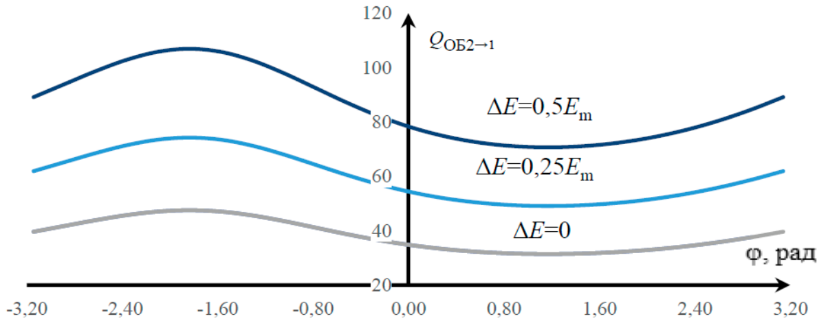
Рисунок 4.8 – Зміна величини обмінної потужності в ЛЕС при зміні параметрів ДРГ
