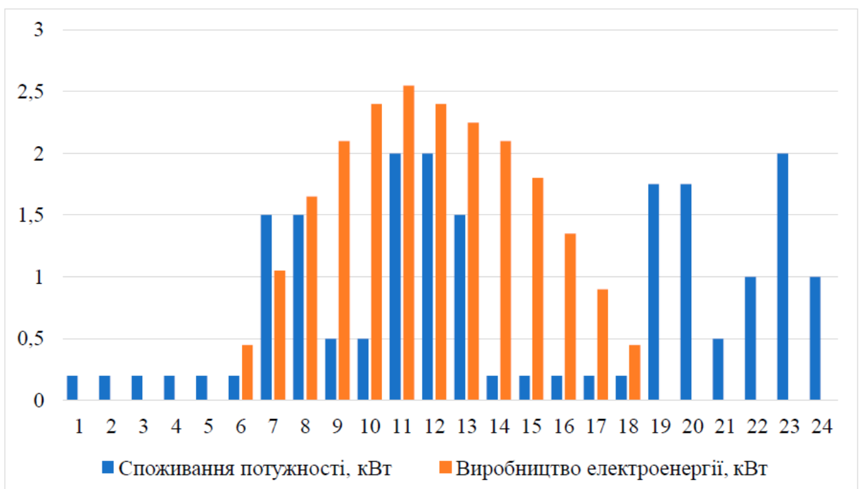
Рисунок 4.1 – Характеристика власного споживання та генерації електроенергії активного споживача
