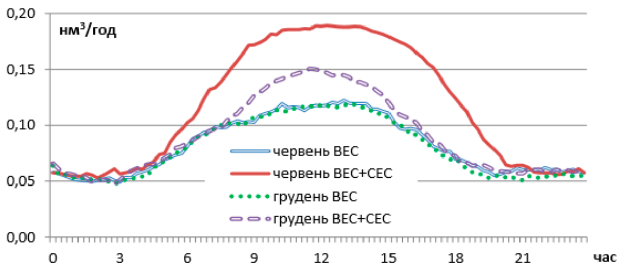
Рисунок 1.6 – Осереднена сумарна потужність ВЕС та СЕС
