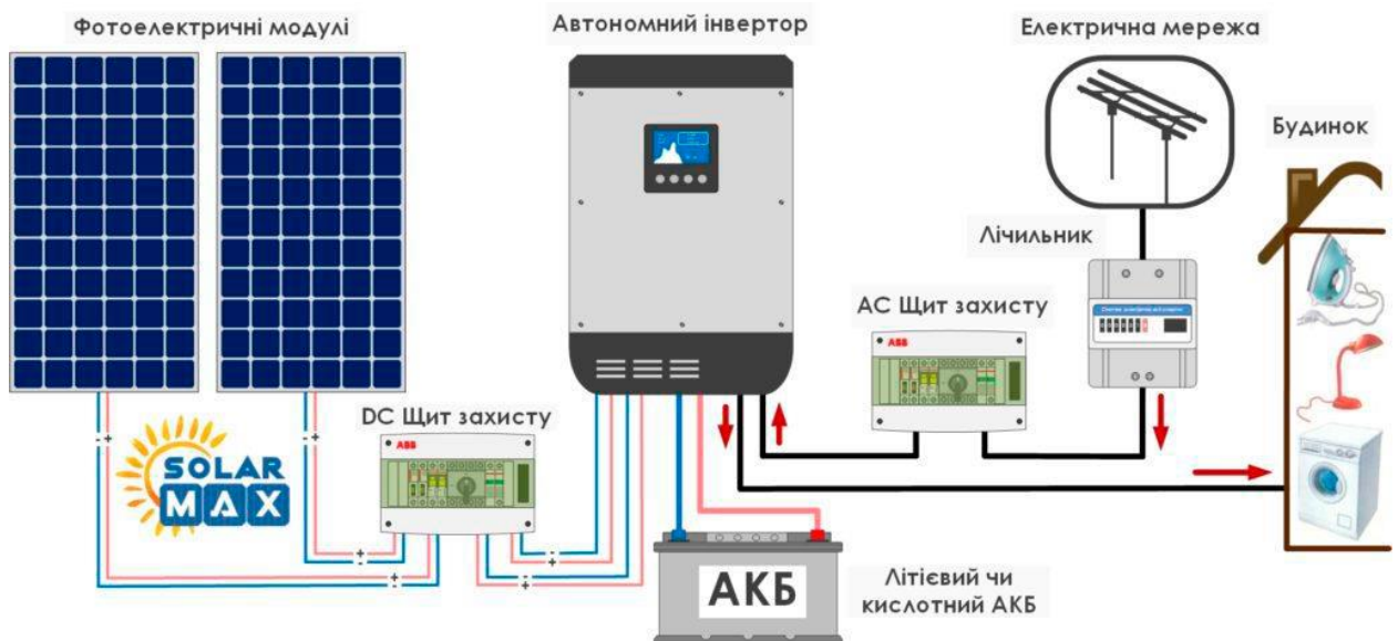
Рисунок 2.5 – Спрощена схема приєднання PV установок та засобів акумулювання електроенергії
