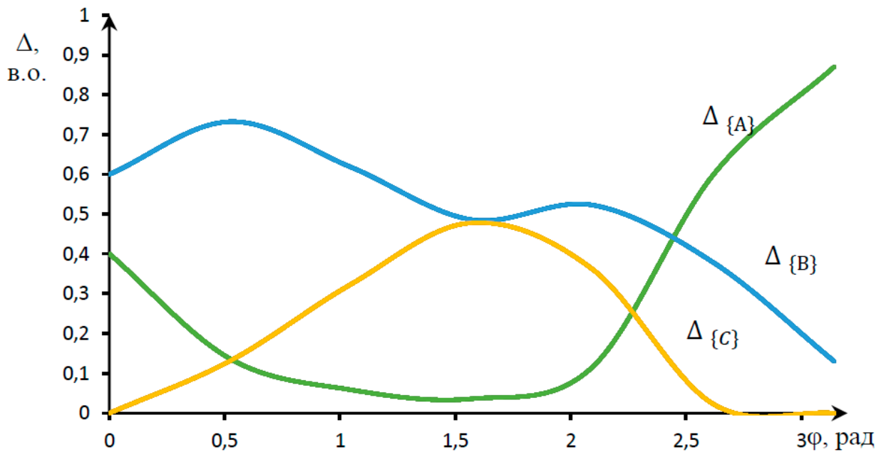
Рисунок 4.10 – Залежність величини обмінної потужності в ЛЕС від зміни кута навантаження
