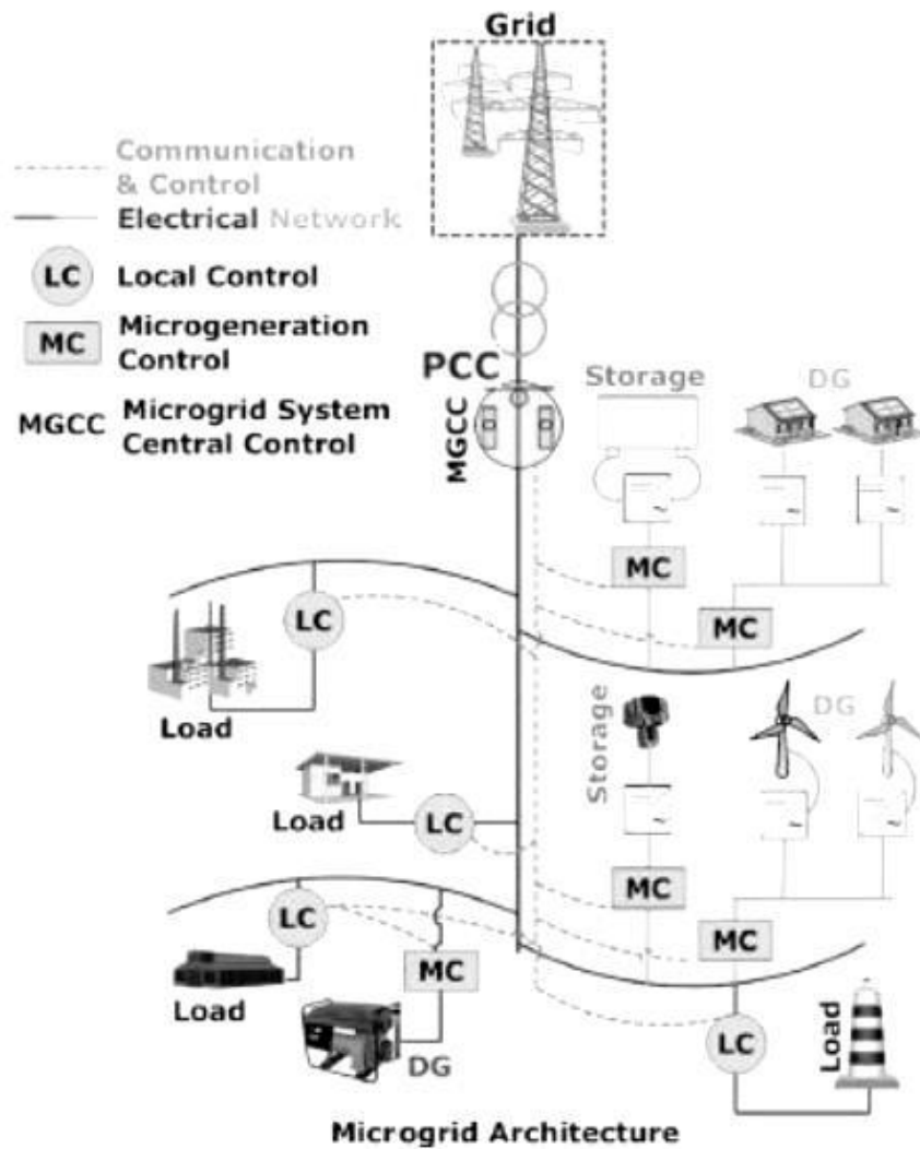
Рисунок 1.1 – Спрощена схема ЛЕС
