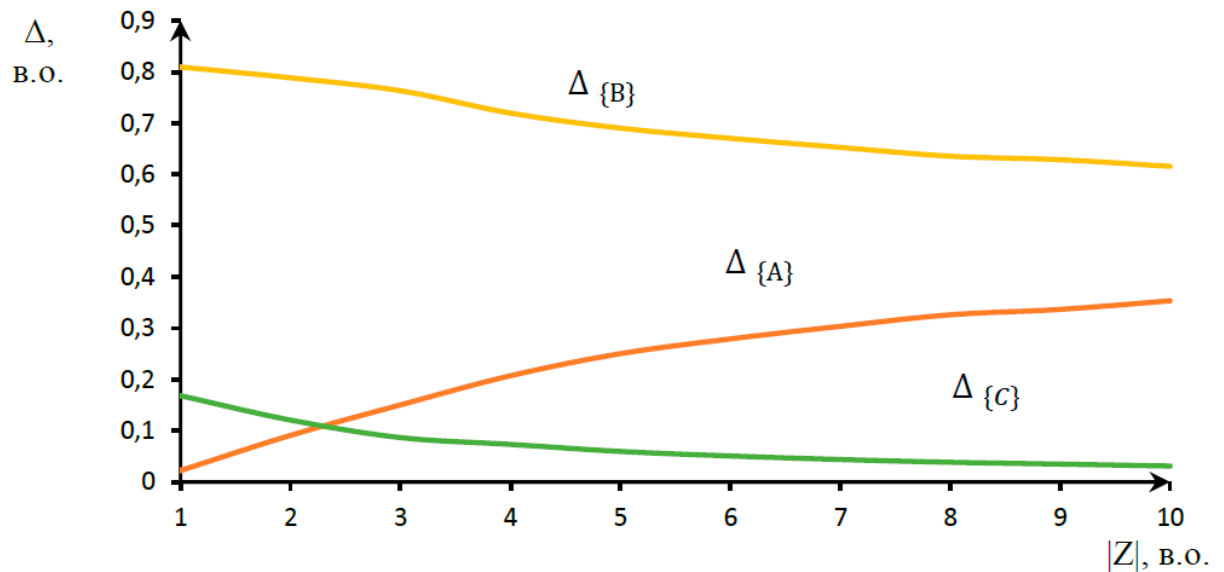
Рисунок 4.9 – Залежність величини обмінної потужності в ЛЕС від зміни модуля навантаження
