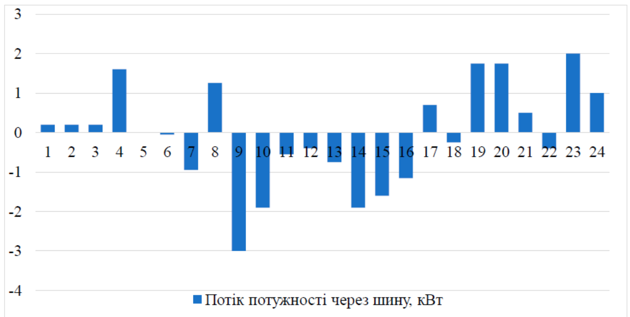
Рисунок 4.3 – Потік потужності через шину активного споживача після застосування алгоритмів керування
