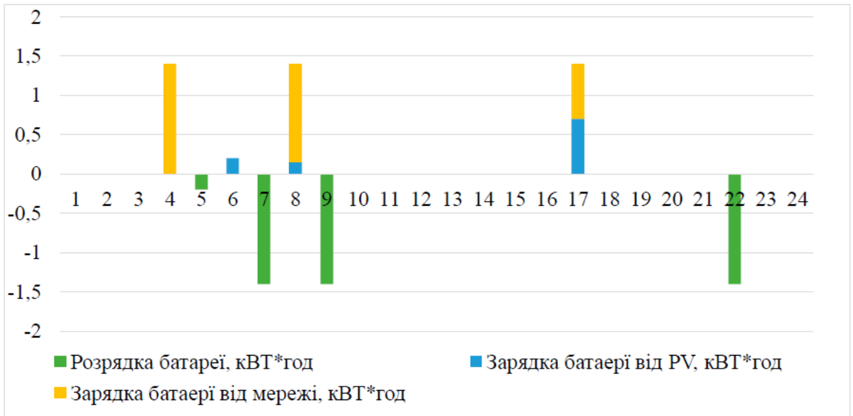
Рисунок 4.4 – Процес зарядження/розрядження батареї
