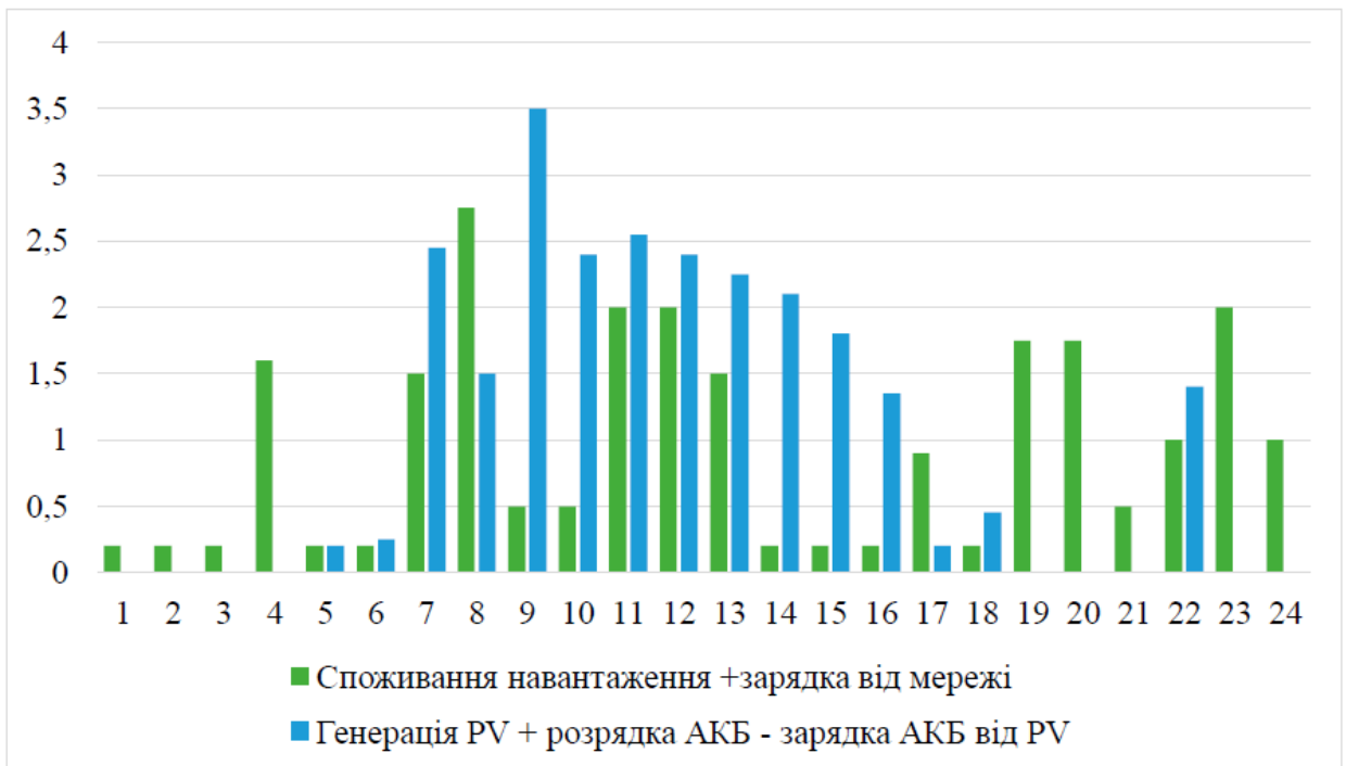
Рисунок 4.5 – Прогнозовані графіки взаємодії активного споживача з мережею
