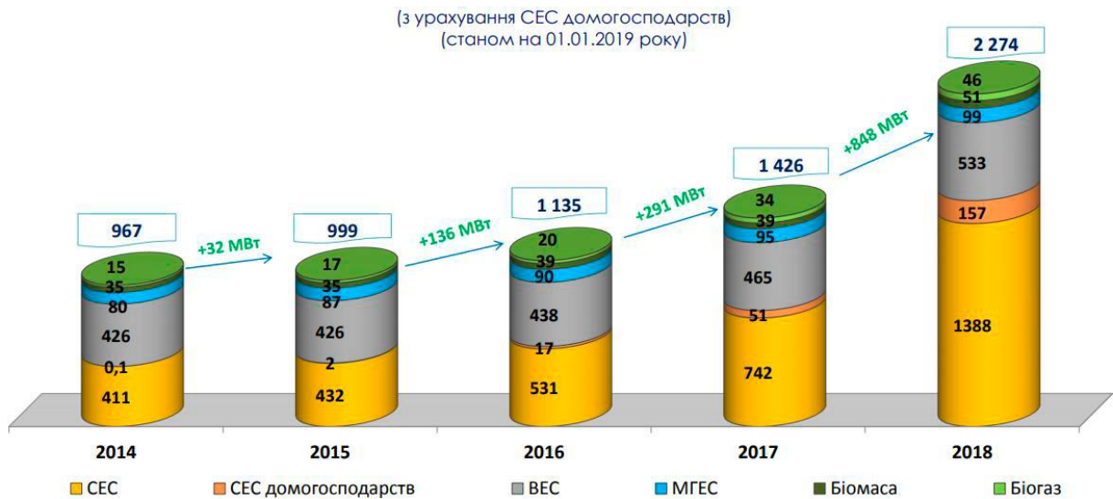
Рисунок 1.5 – Встановлена потужність об'єктів відновлювальної енергетики, що працюють за “зеленим” тарифом в Україні
