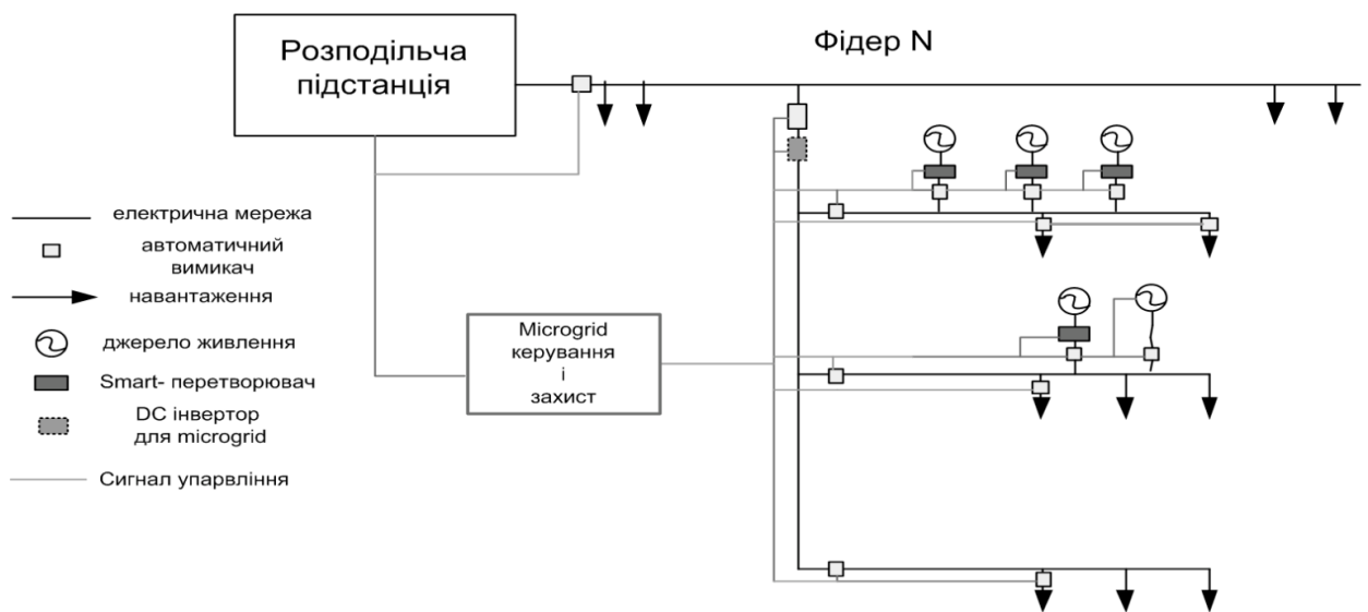
Рисунок 1.2 – Кінцева схема еволюції ЛЕС
