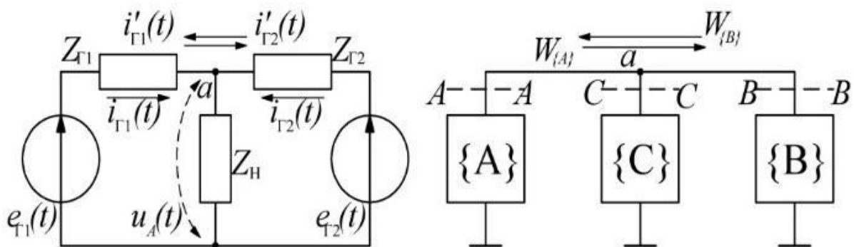
Рисунок 4.7 – Схема ЛЕС з двома генераторами та спільним навантаженням
