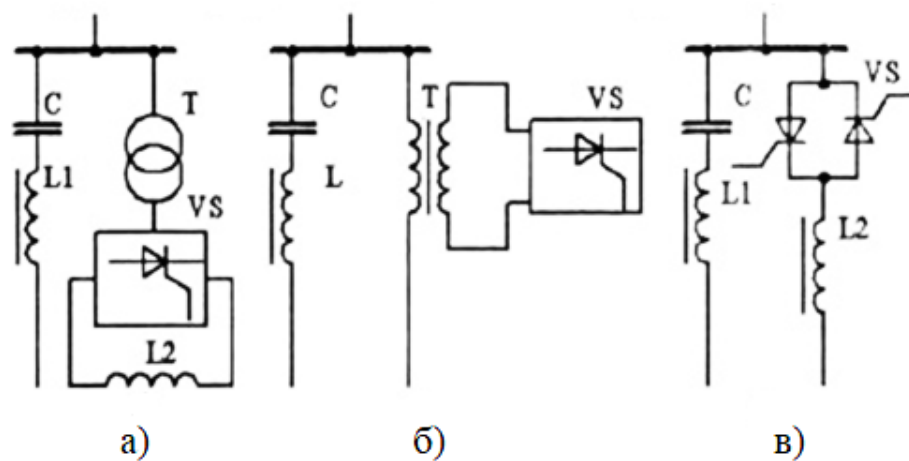
Рисунок 3.4 – Електричні схеми статичних компенсуючих установок:
