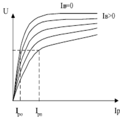
Рисунок 3.6 – Характеристики реактора з підмагніченням I_B - струм підмагнічення
