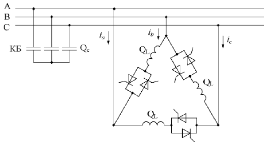
Рисунок 3.10 – Принципова схема компенсатора з реакторами, керованими вентилями
