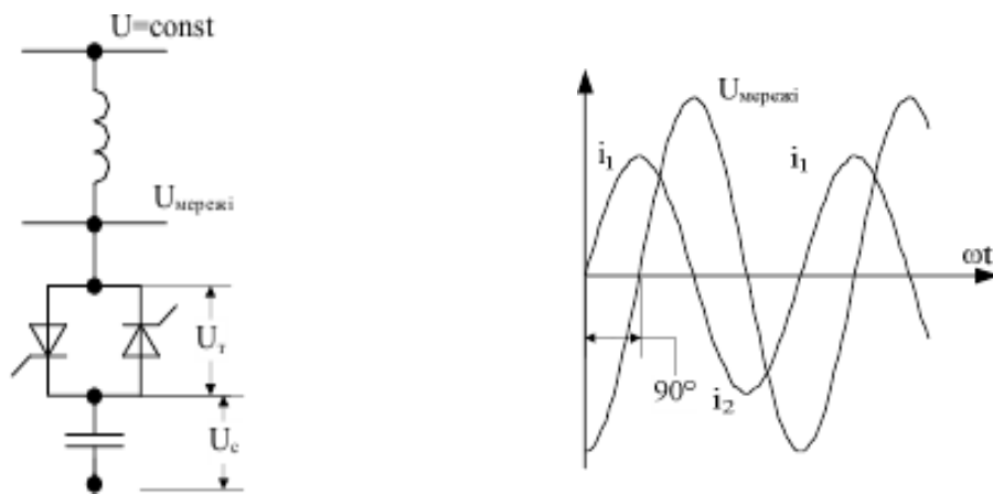
а) принципова схема однієї фази
