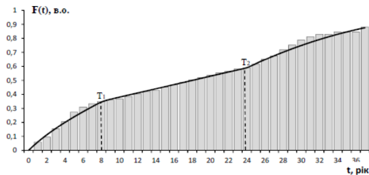
Рисунок 2.4 – Статична функція розподілу відмов повітряних вимикачів
