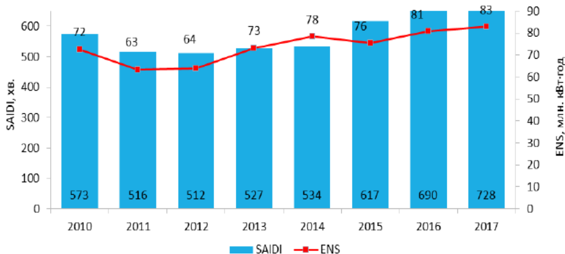
Рисунок 2.2 – Динаміка фактичних показників SAIDI та ENS по Україні
