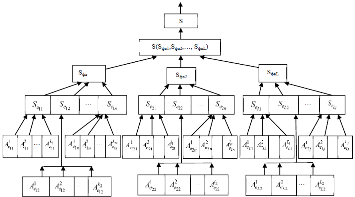
Рисунок 2.5 - Загальна ієрархічна структурна схема моделі визначення показника відновлення ресурсу електрообладнання: A_i – параметри технічного стану після ремонту електрообладнання; S_e – ресурс працездатності після ремонту елементів електрообладнання; S_{\phi_{\text{в}}} – ресурс працездатності після ремонту функціональних вузлів електрообладнання
