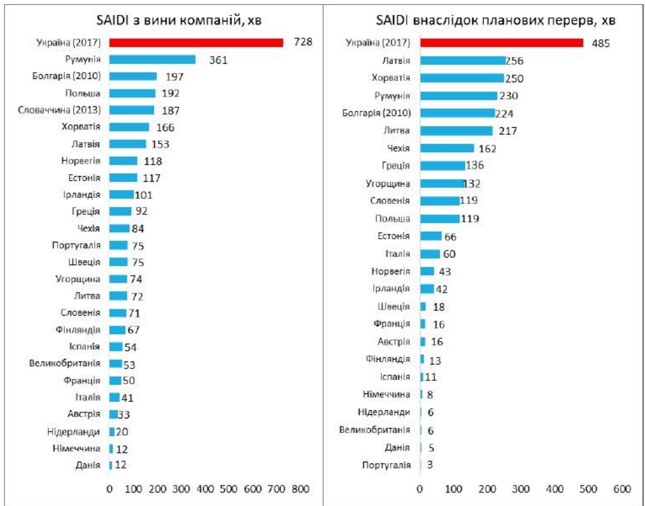
Рисунок 2.3 – Показники SAIDI країн Європи та України
