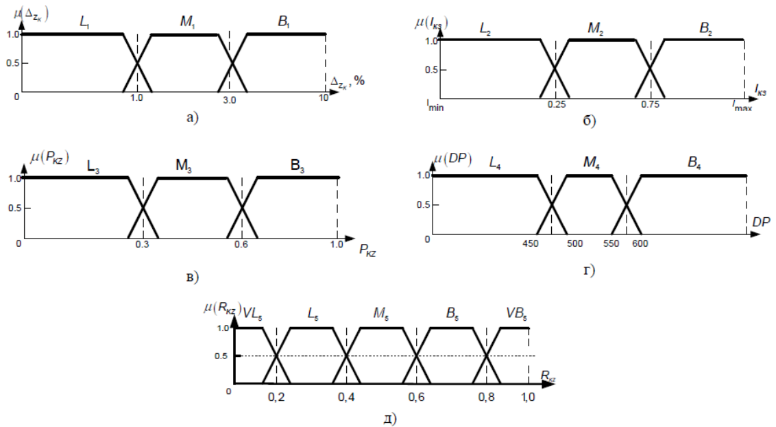
Рисунок 2.8 – Функції належності терм-множин вхідних і вихідної лінгвістичної змінних: а) – змінення опору КЗ; б) – величина наскрізного струму КЗ; в) – імовірність наскрізного струму в обмотках СТ; г) – ступінь полімеризації ізоляції; д) – ризик відмови СТ при дії струмів зовнішніх КЗ
