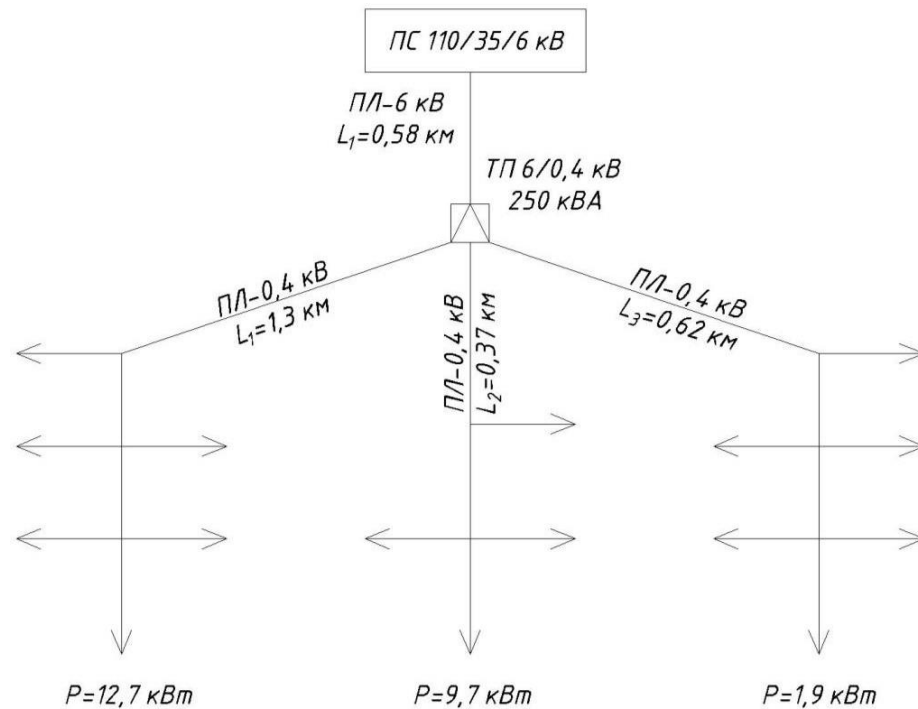
Рисунок 6 – Існуюча схема електропостачання в Гніванському вузлі
