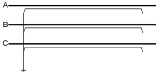
Рисунок 3.1 – Схема заземлення екранів з одного кінця
