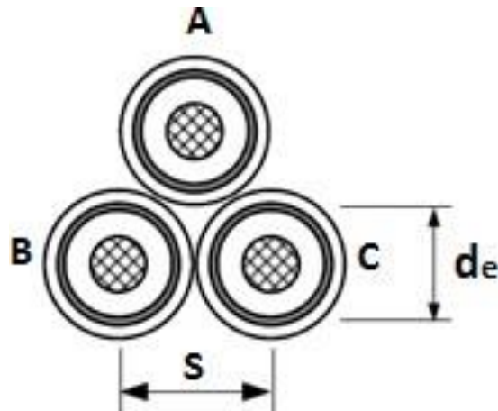
Рисунок 3.3 - Прокладка трифазної групи однофазних кабелів у вигляді зімкненого трикутника
