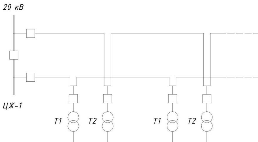
Рисунок 2.8 – Вдосконалена двопротенева схема
