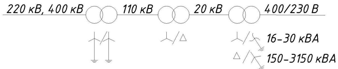
Рисунок 1.1 – Схема передачі енергії і режими заземлення нейтралі силових трансформаторів, використувана в Фінляндії
