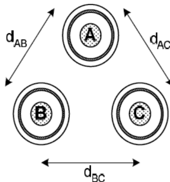
Рисунок 2.3 - Розташування однофазних кабелів в вершинах трикутника
