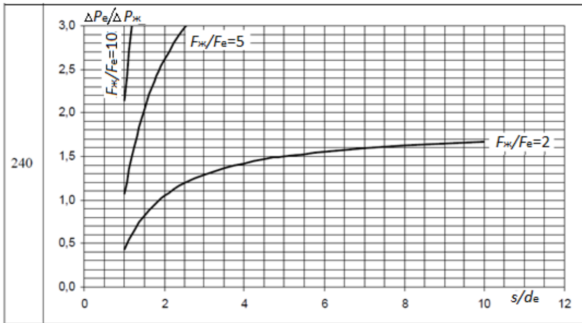
Рисунок 3.12 - Втрати в екранах кабелів в залежності від перерізу екрана 240 мм 2
