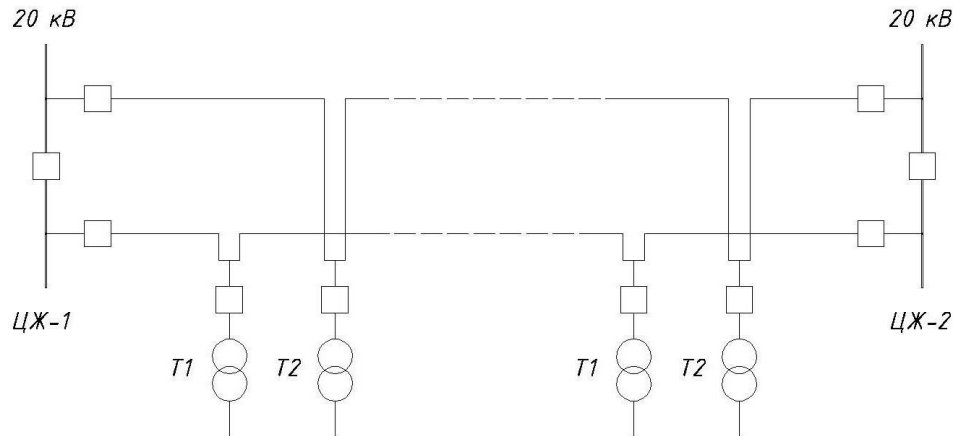
Рисунок 2.7 – Типова двопротенева схема
