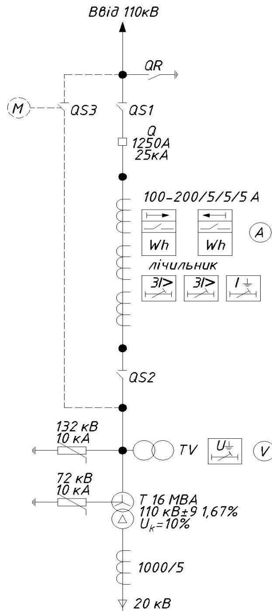
Рисунок 1.2 – Однолінійна схема однострансформаторної підстанції 110/20 кВ
