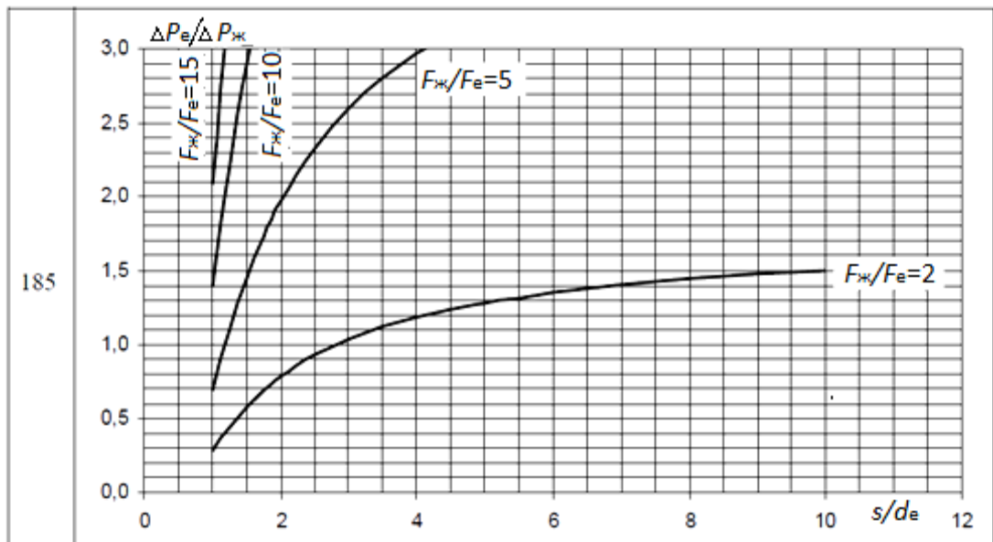
Рисунок 3.11 - Втрати в екранах кабелів в залежності від перерізу екрана 185 \text{ мм}^2
