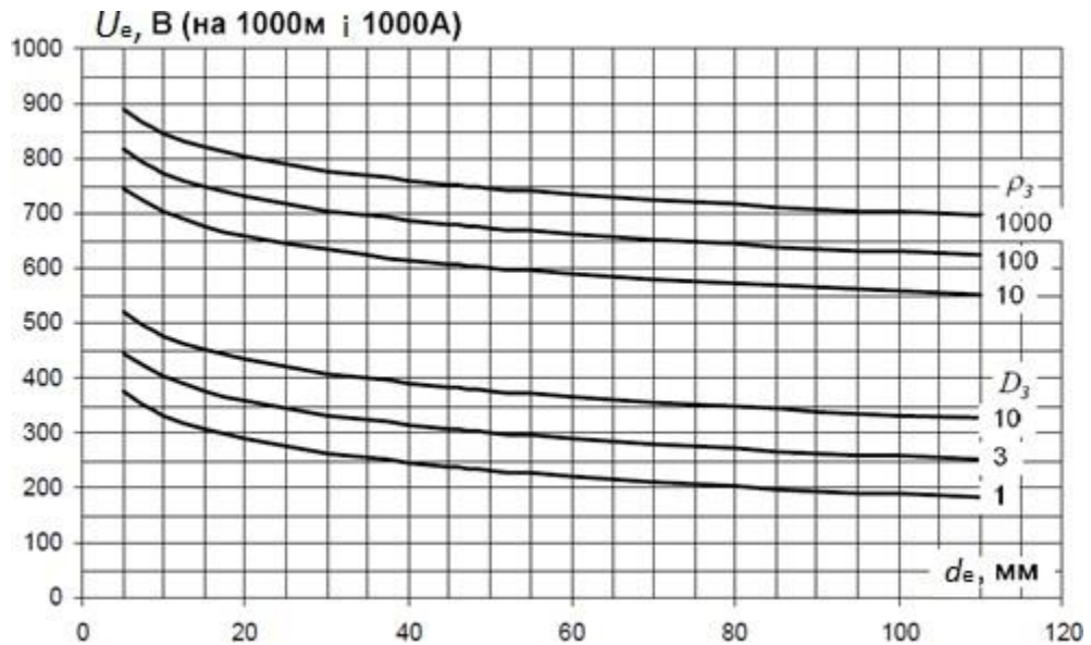
Рисунок 3.13 – Напруга на екрані кабелю відносно землі для розрахунку по (1), (6), (7) в залежності від співвідношення s/d_\epsilon для кабелю довжиною 1000 м при струмі 1000 А
