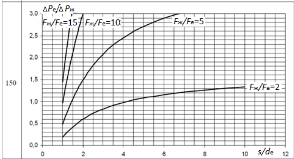
Рисунок 3.10 – Втрати в екранах кабелів в залежності від перерізу екрана 150 \text{ мм}^2
