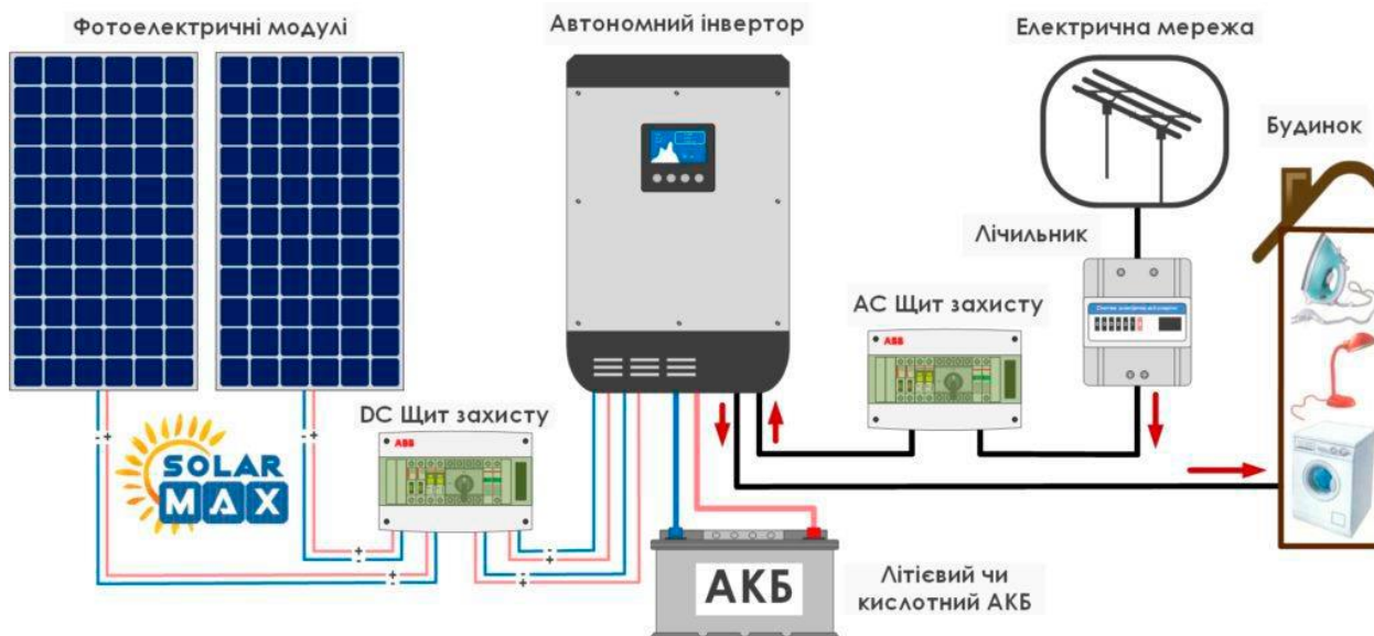
Рисунок 2.5 – Спрощена схема приєднання PV установок та засобів акумулювання електроенергії
