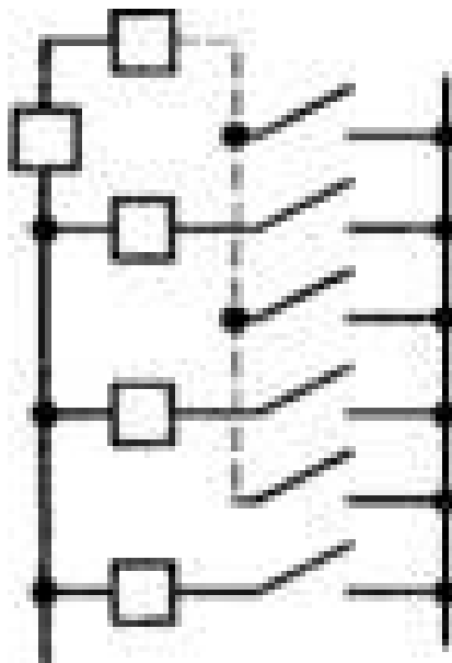
Рисунок 1.5 – Змішана схема електропостачання:
