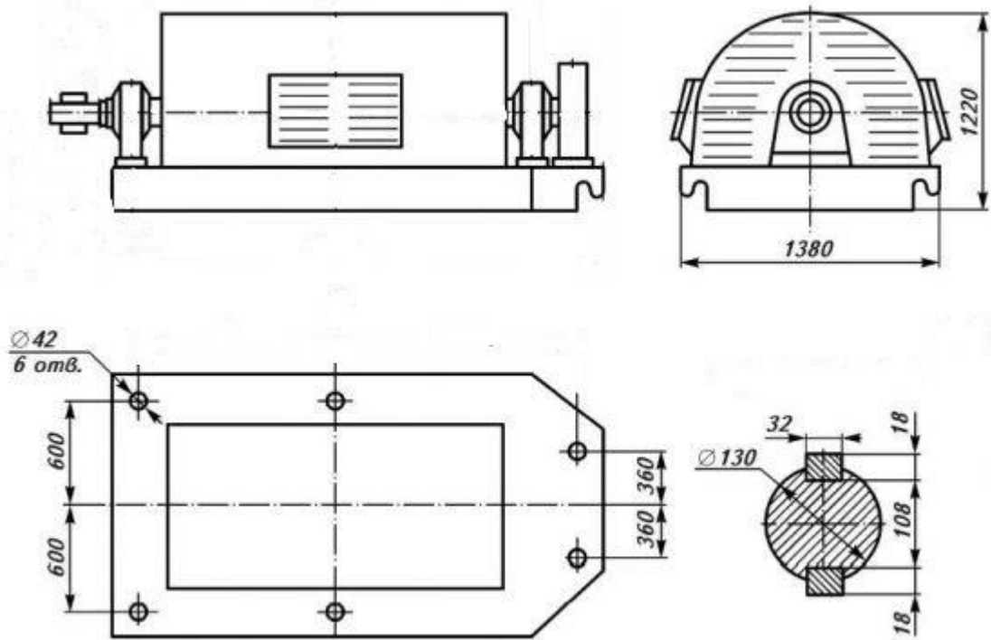
Рисунок 3.6 – Синхронний двигун типу СТДМП4000-2
