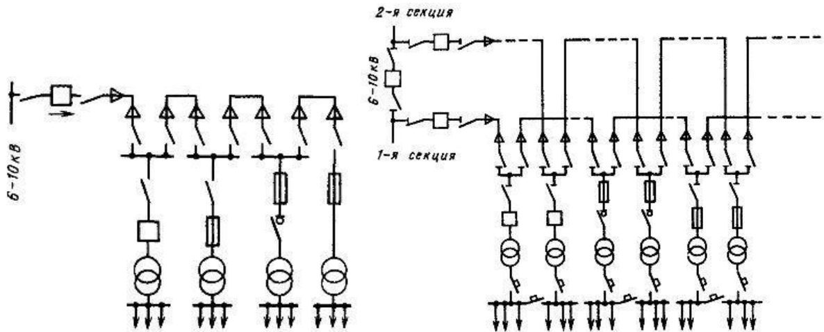
Рисунок 1.3 – Приклади магістральної схеми електропостачання
