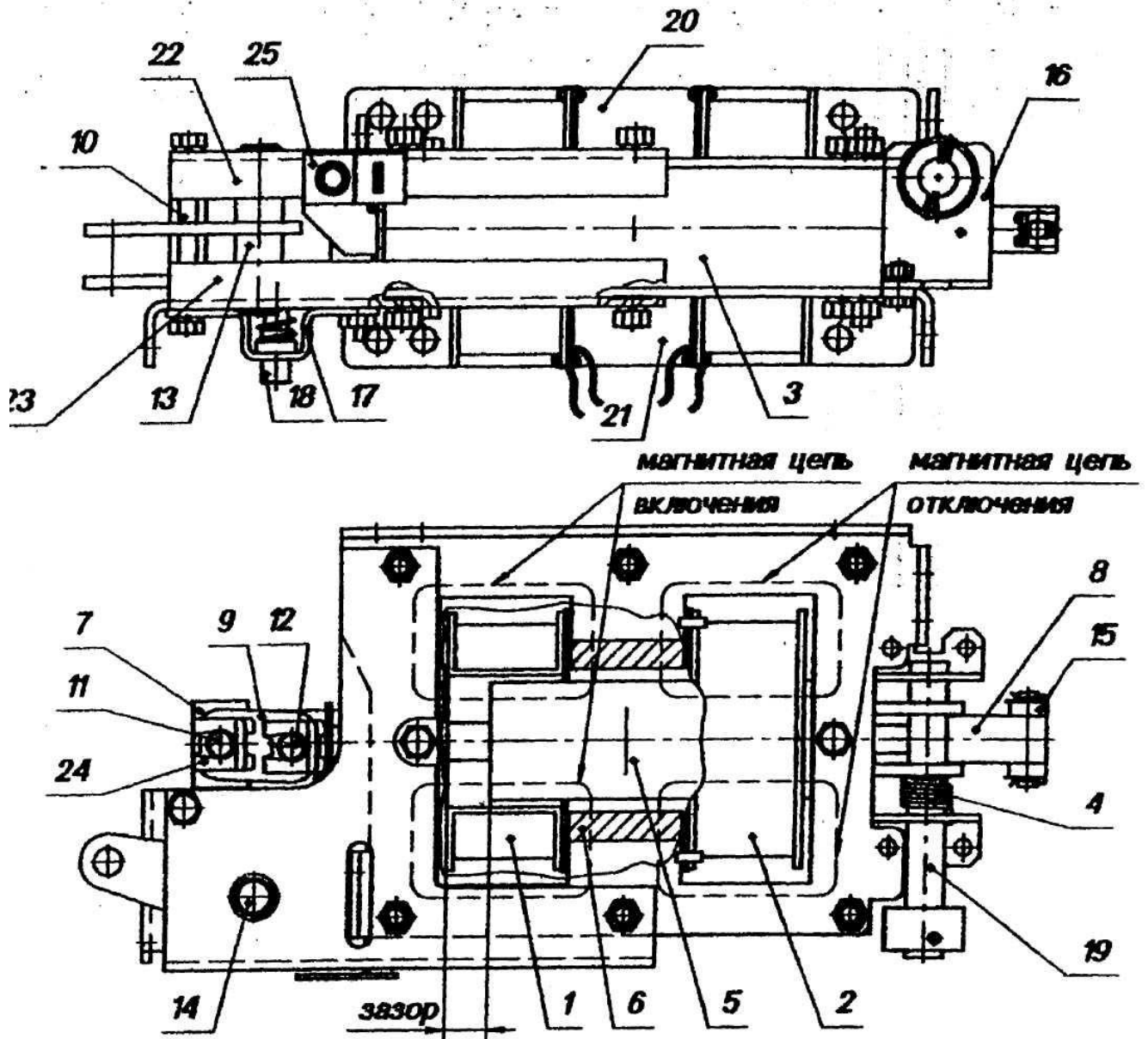
Рисунок 3.3 – Электромагнит вимикача
