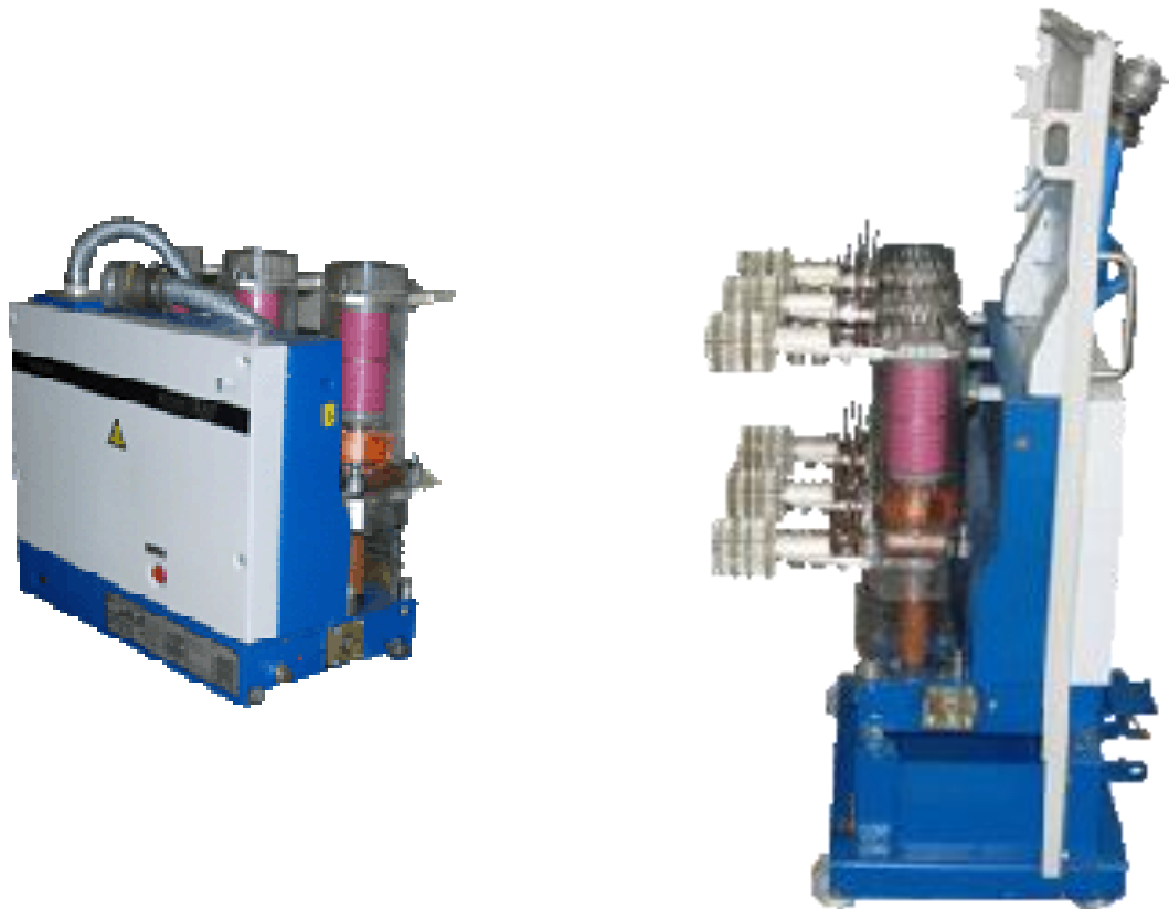
Рисунок 2.3 – Вакуумний вимикач ВБУЭ(П)3 – 10 – 20/1000У2
