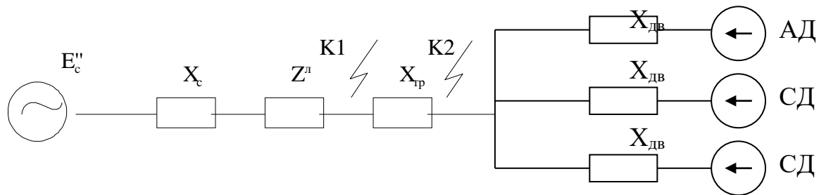
Рис. 2.4 Схема заміщення (точка К1)
