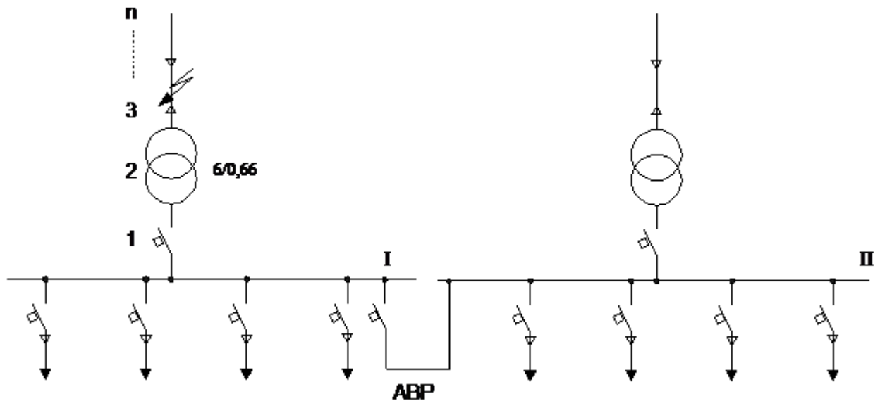
Рис. 5.3 Принципова схема електропостачання секції шин I
