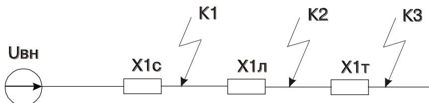
Рис. 4.2 Схема заміщення прямої послідовності
