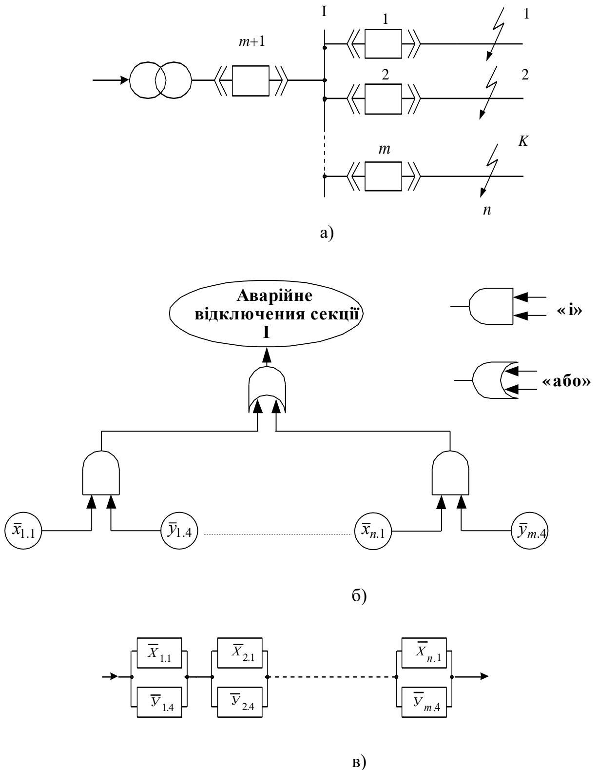
Рис. 5.2 Приклад схеми
