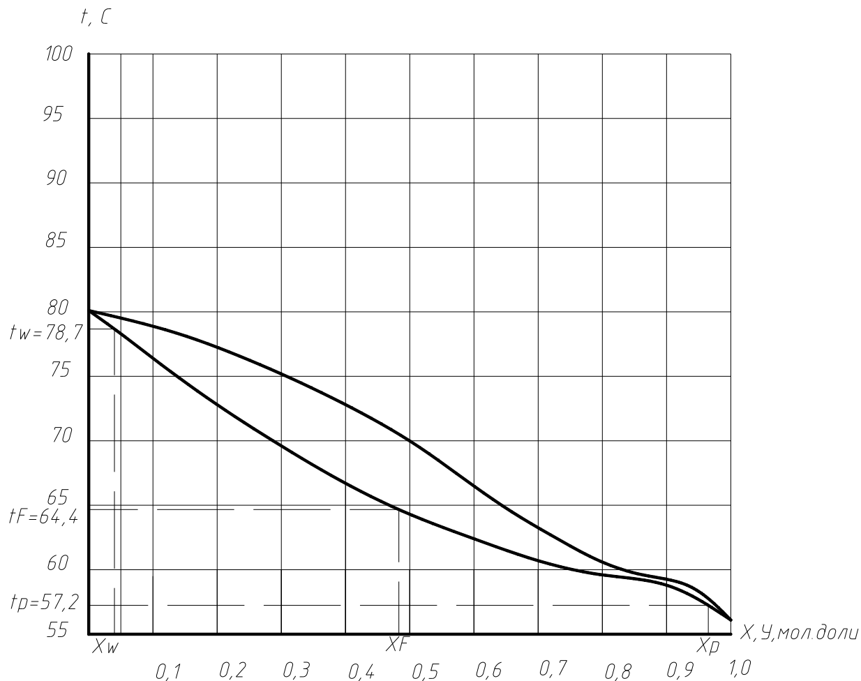
Рисунок 4.2 - Ізобару температур кипіння й конденсації
