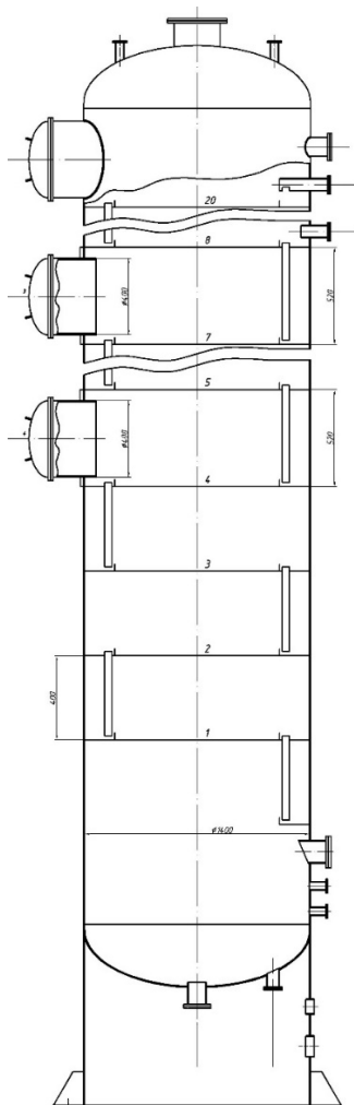
Рисунок 2.2 – Колона з сітчастими тарілками
