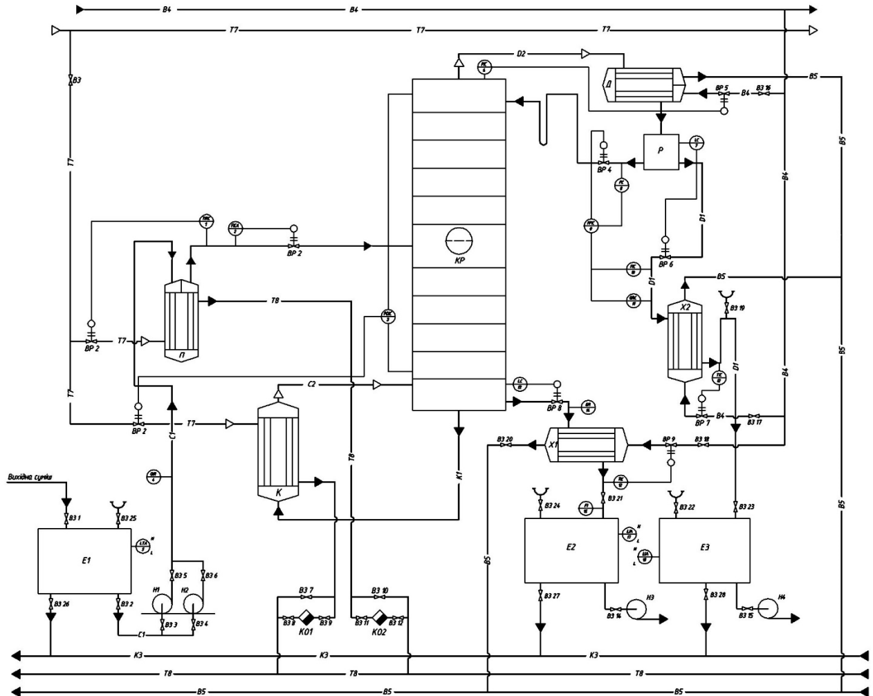
Рисунок 2.1 – Схема ректифікаційній установки
