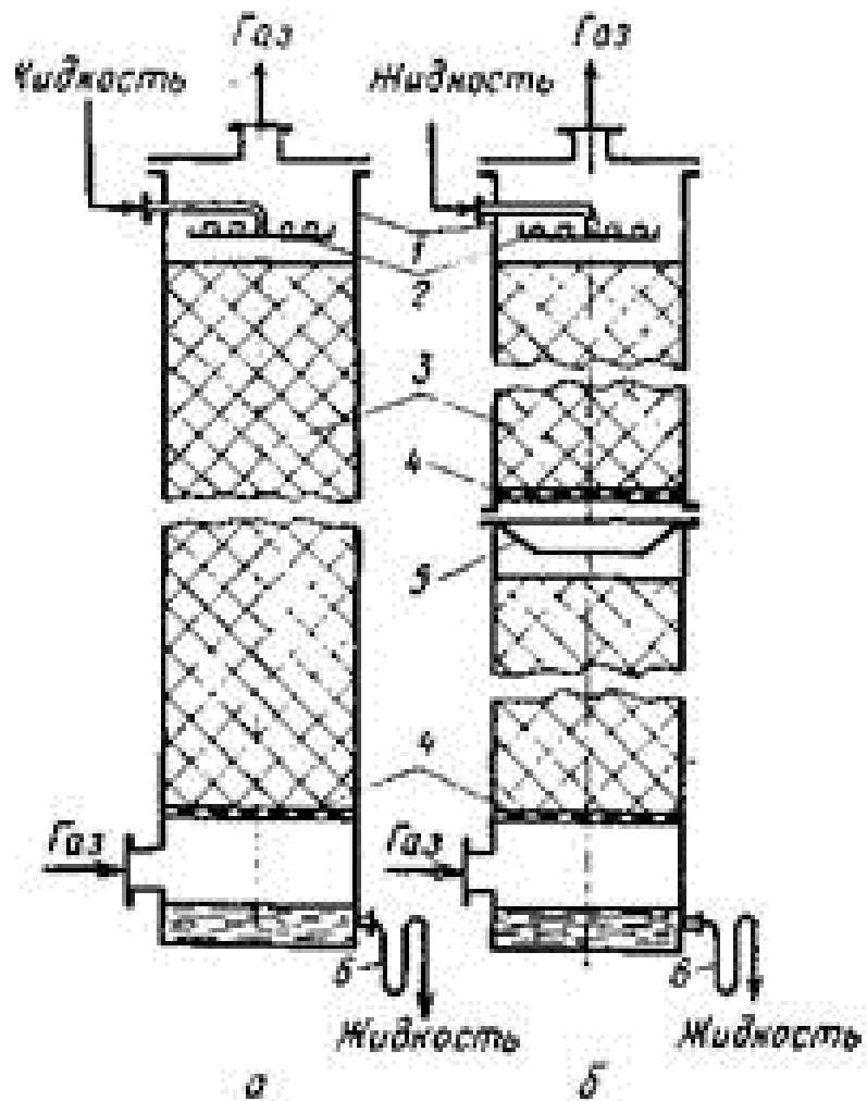
Рисунок 2.2 – Насадочна колона.
