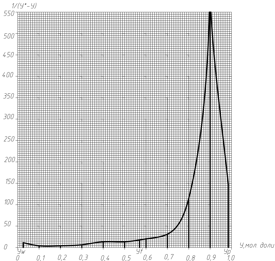
Рисунок 4.4 - До визначення числа одиниць переносу (ЧОП).
