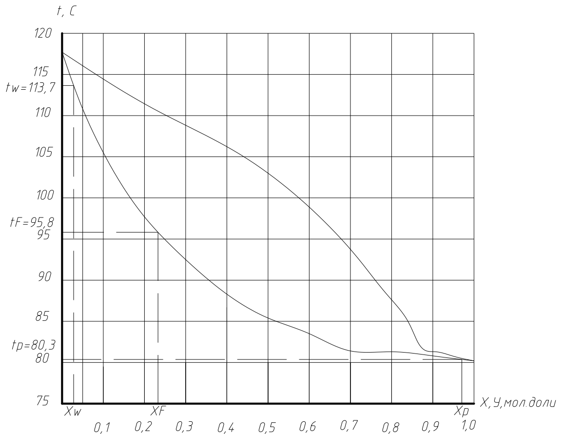
Рисунок 4.2 - Ізобару температур кипіння й конденсації
