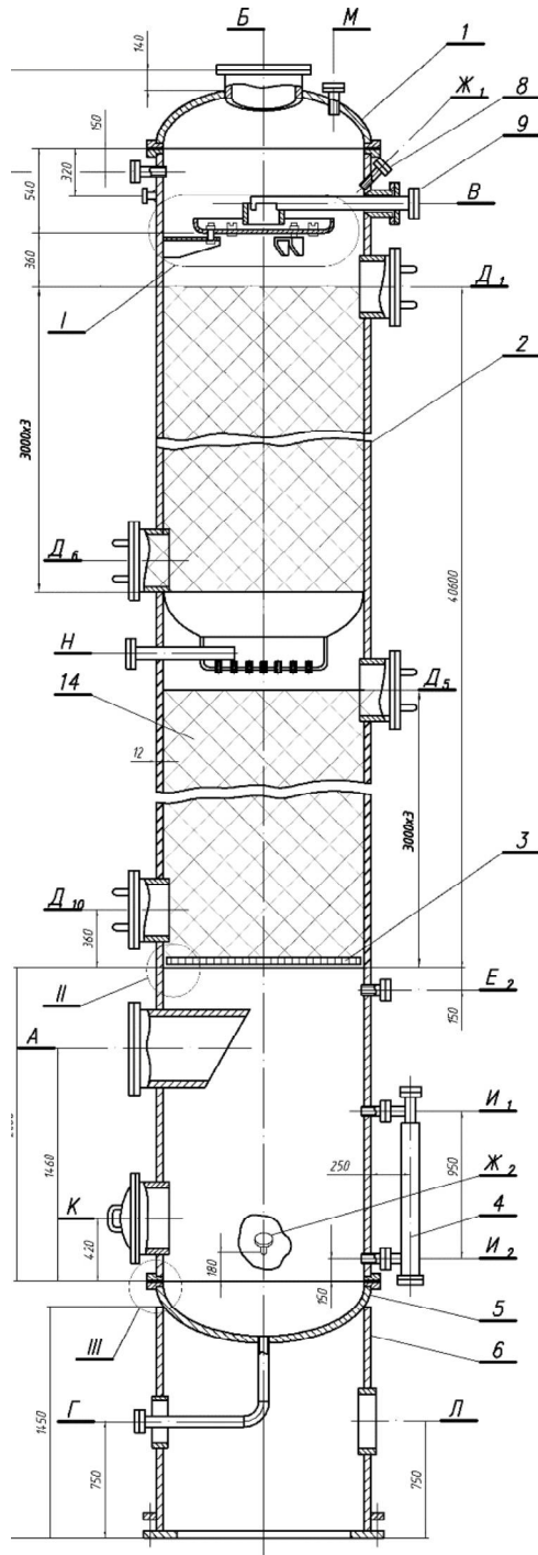
Рисунок. 2.2 – Насадочна колона
