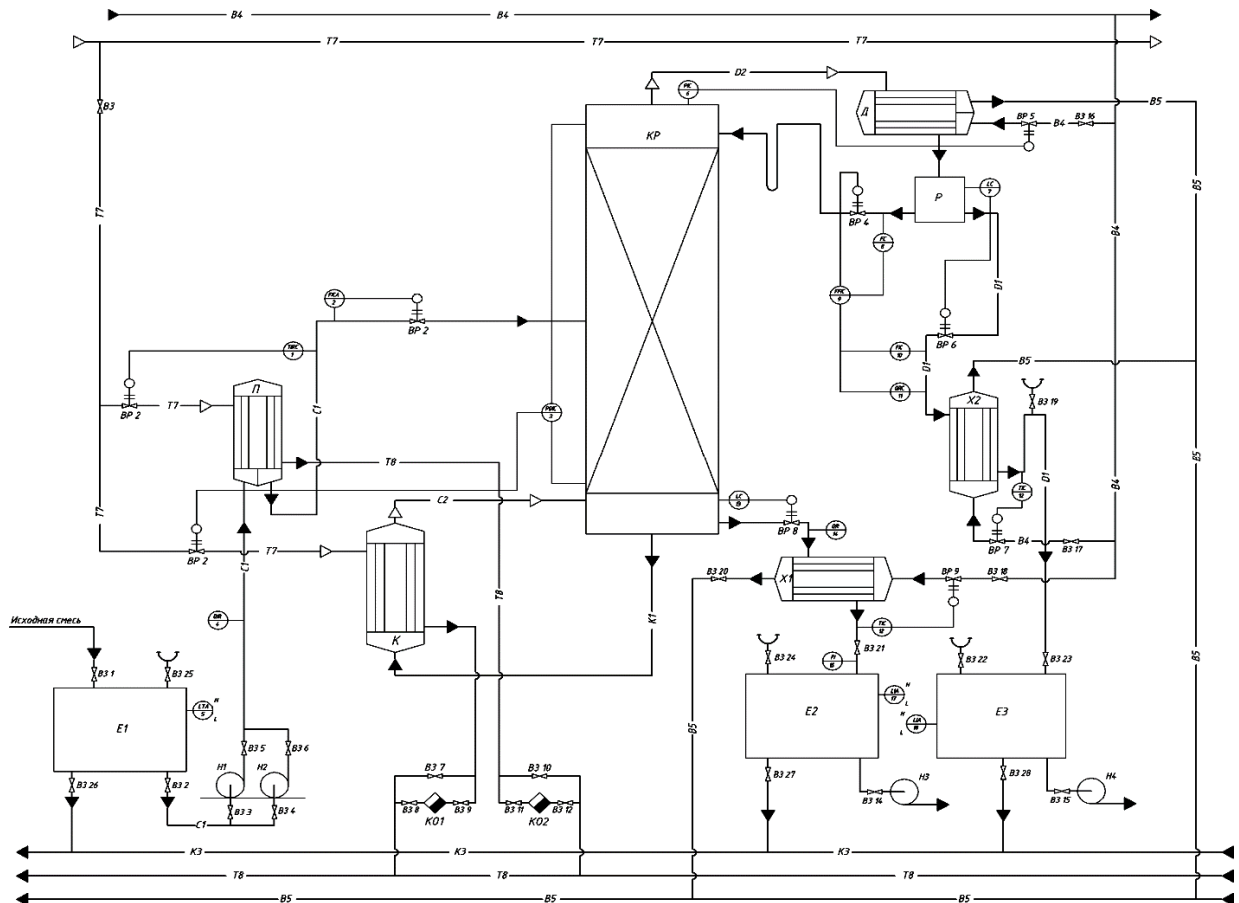
Рисунок. 2.1 – Схема ректифікаційної установки
