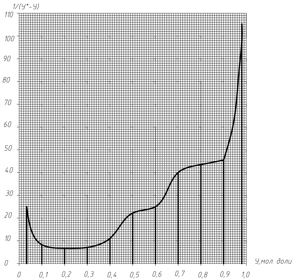
Рис. 4.4 - До визначення числа одиниць переносу.
