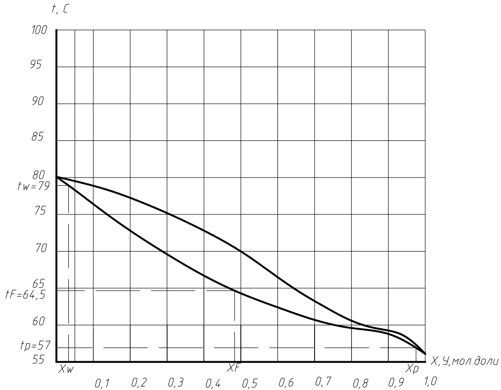
Рис. 4.2 - Ізобару температур кипіння й конденсації.
