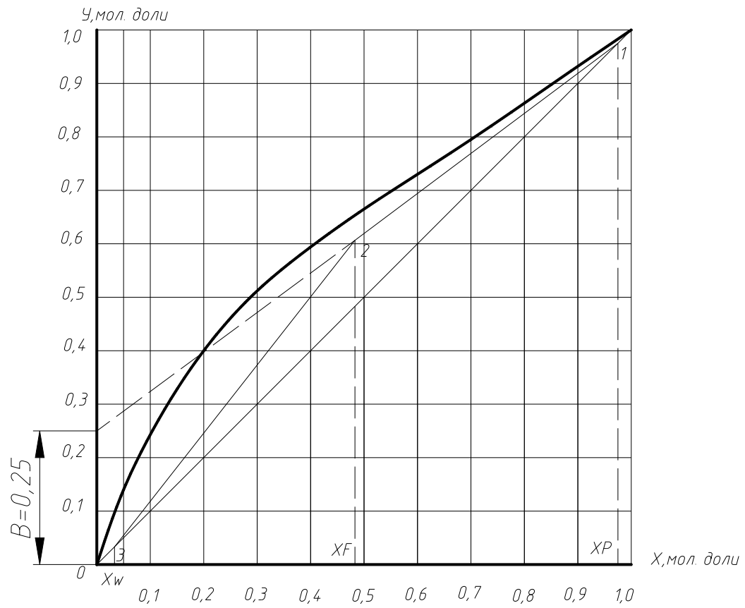
Рис. 4.3 - Побудова робочих ліній.
