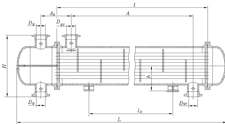
Рисунок 2.3 – Кожухотрубчатий теплообмінний апарат (дефлегматор)
