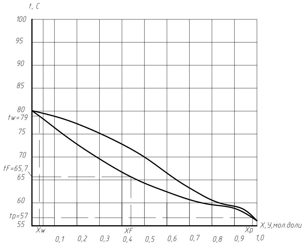
Рис. 4.2 – Ізобару температур кипіння й конденсації.
