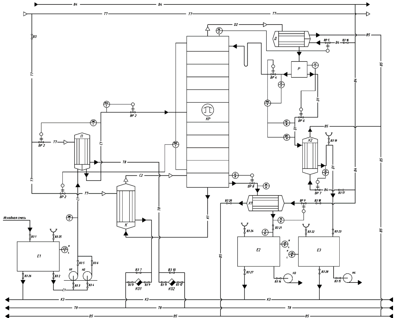
Рисунок 2.1 – Схема ректифікаційній установці
