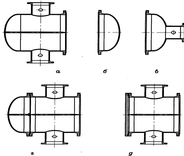
Рис. 6.1 – Типові конструкції розподільних камер і кришок
