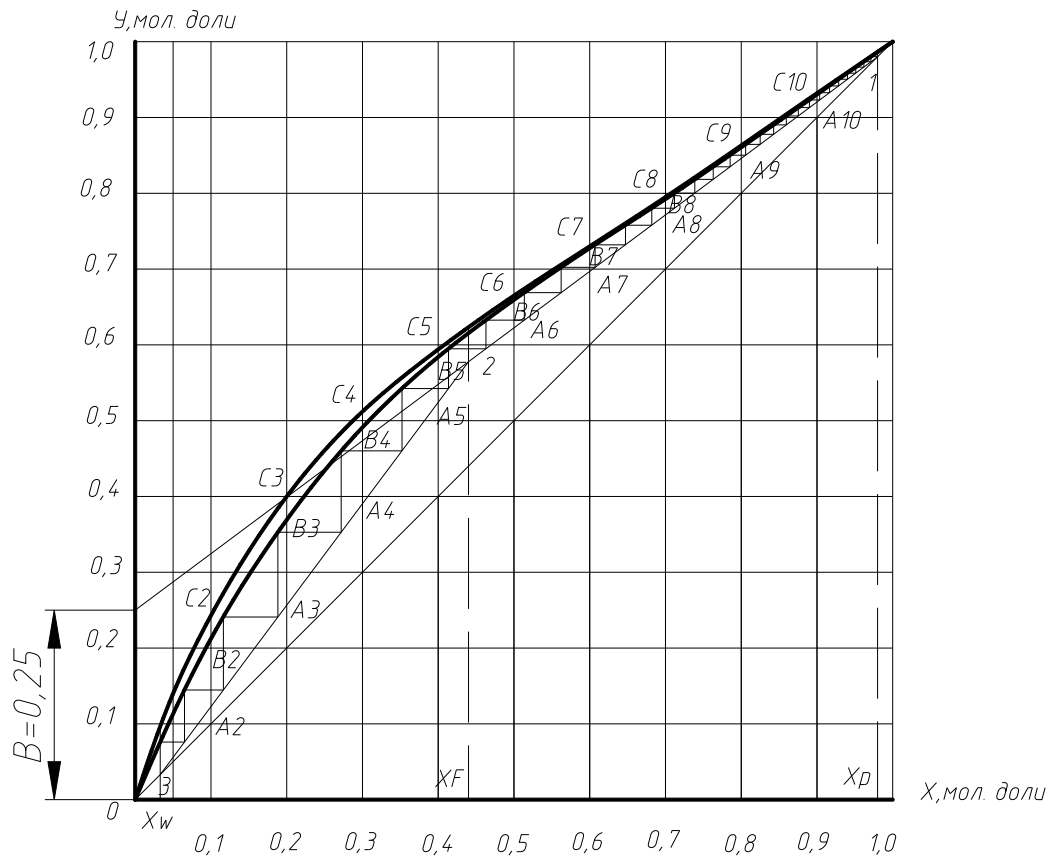
Рис. 4.3 – Побудова кінетичної кривій і визначення числа дійсних тарілок (у масштабі 1:1).
