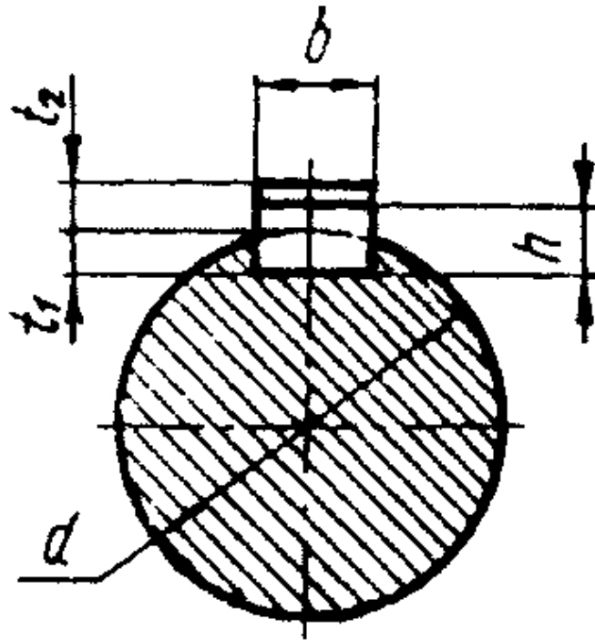
Рисунок 6.4 - Схема шпонкового з'єднання
