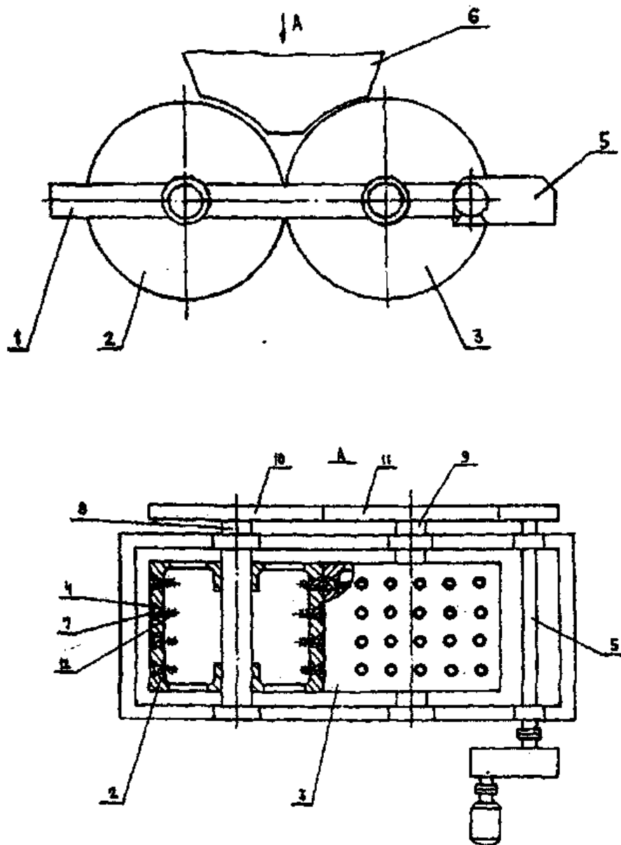
Рисунок 3.1 - Брикетні прес - вальці удосконаленої конструкції
