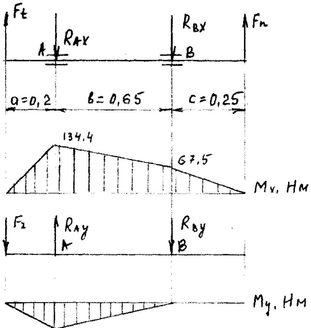
Рисунок 6.3 - Розрахункова схема та епюри згинання для вала
