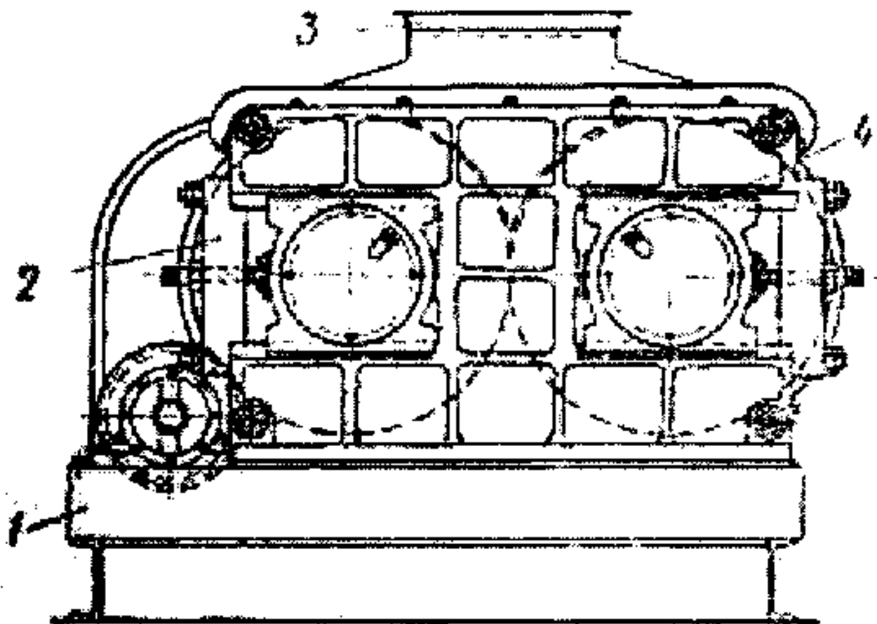
Рисунок 3.1 - Прес-вальці:
